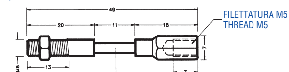
MOLLA DI DISASSAMENTO DISASSAMENTO MAX 3 mm
